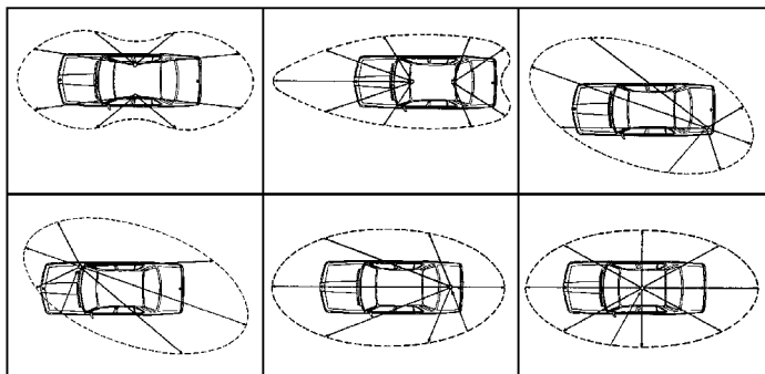
ANTENNENKEULE
