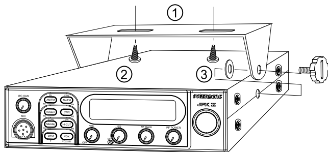
ALLGEMEINER MONTAGEPLAN
